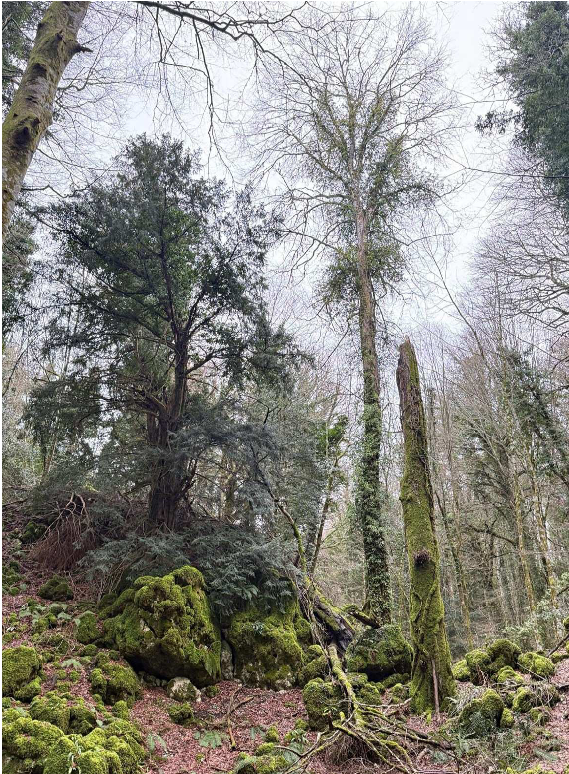
Figura 4. Situazione caratterizzata da elevata eterogeneità morfologica e strutturale. La compresenza di necromassa in piedi e a terra con differenti stadi di decomposizione, stratificazione verticale della vegetazione e discontinuità del substrato.
